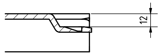
A-A ( 1 : 2 )
